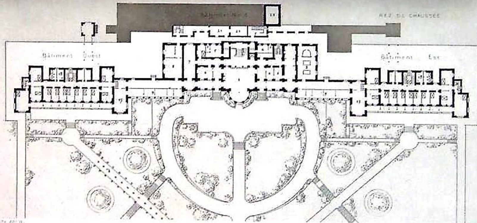
ETABLISSEMENT DU MONT DES OISEAUX BORDAUX Plans du Rez de Chaussée et du 1 er étage
